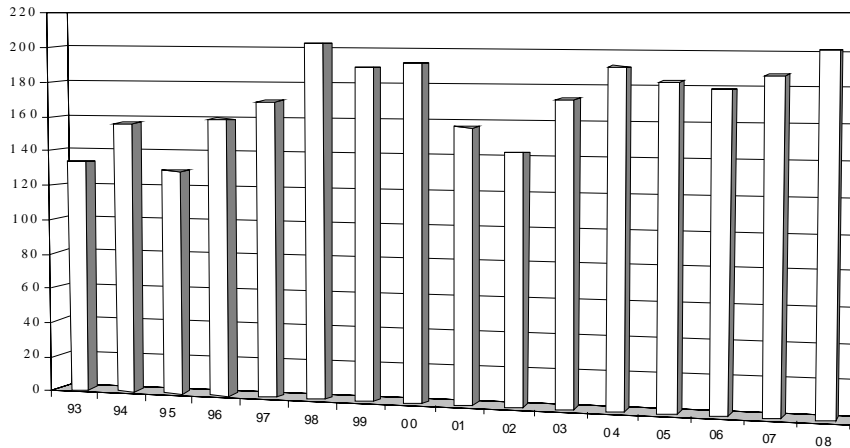
Galvanikschlammfall 1993 - 2008 [t]
