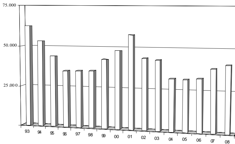
Abwasseranfall 1993 - 2008 [m³]
